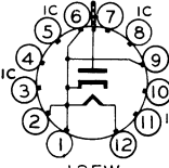
12EW 2AS2
