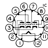
12BQ 6C10
