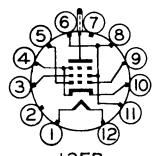
12FB 6HF5
