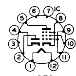
12FC 33GT7
