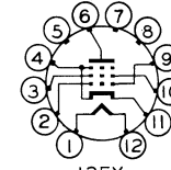
12EY 6HE5
