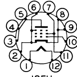
12EU 7984, 8156
