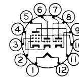
12CA 6M11
