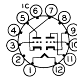
12BM 6FJ7
