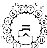
12DQ 2AH2
