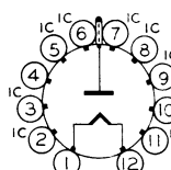
12DQ 1AD2
