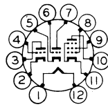
12FP 6BH11
