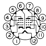
12BW 6J11
