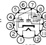
12FT 23Z9
