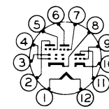
12ER 6BA11
