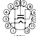
12EX 3AT2
