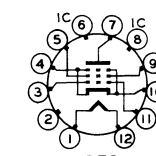
12ES 6HD5
